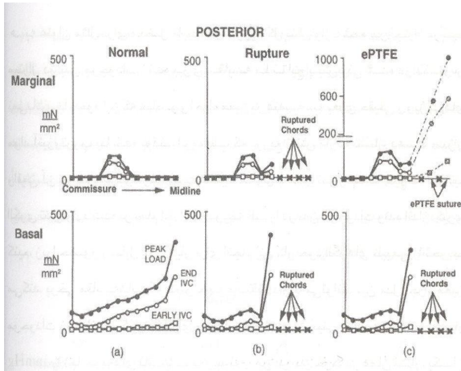
تصویر ۸- سطوح فشار بر روی طناب وتری لت خلفی درجه میترال در سه زمان (ابتدای مرحله بارگیری، مرحله انقباض ایزولولمیک و اوج بارگیری‌ها: (a) مدل نرمال، (b) مدل دچار پارگی طناب وتری و (c) مدل دارای جایگزینی ePTFE
